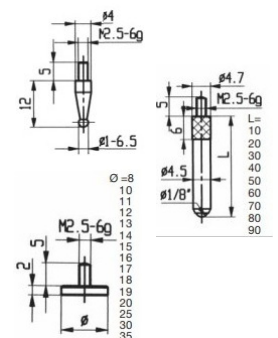
OPTIONAL ANVILS
